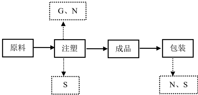
图 2-2 项目塑料盒生产工艺流程及产排污环节图
