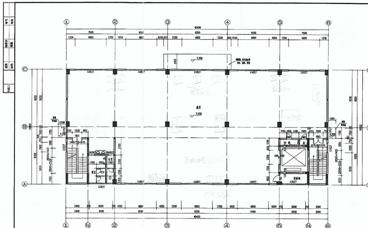
二层平面图 1:100
