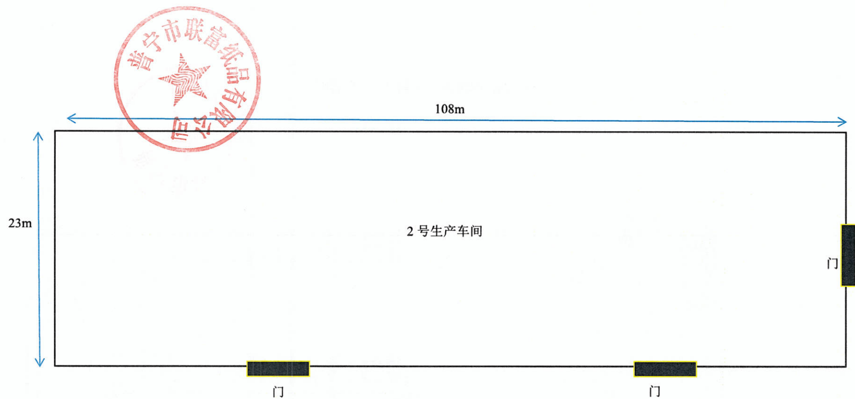
附图 3-3 2号生产车间平面布置图
