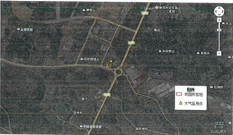
附图 1 项目大气监测布点图
