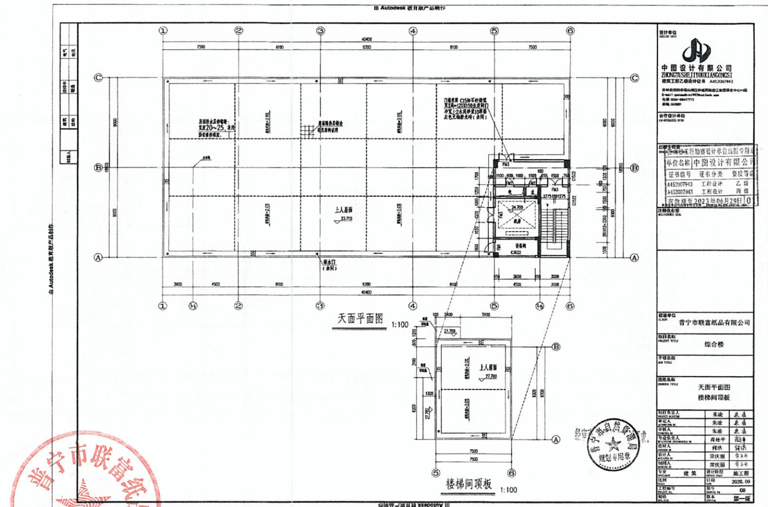
附图 3-1 综合楼平面布置图
