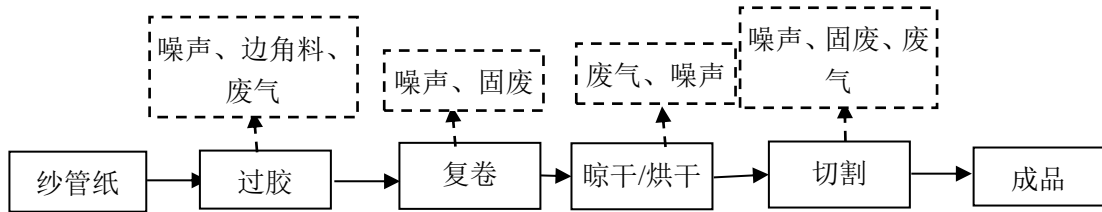
图 2-1 项目纸筒生产工艺流程及产污环节
