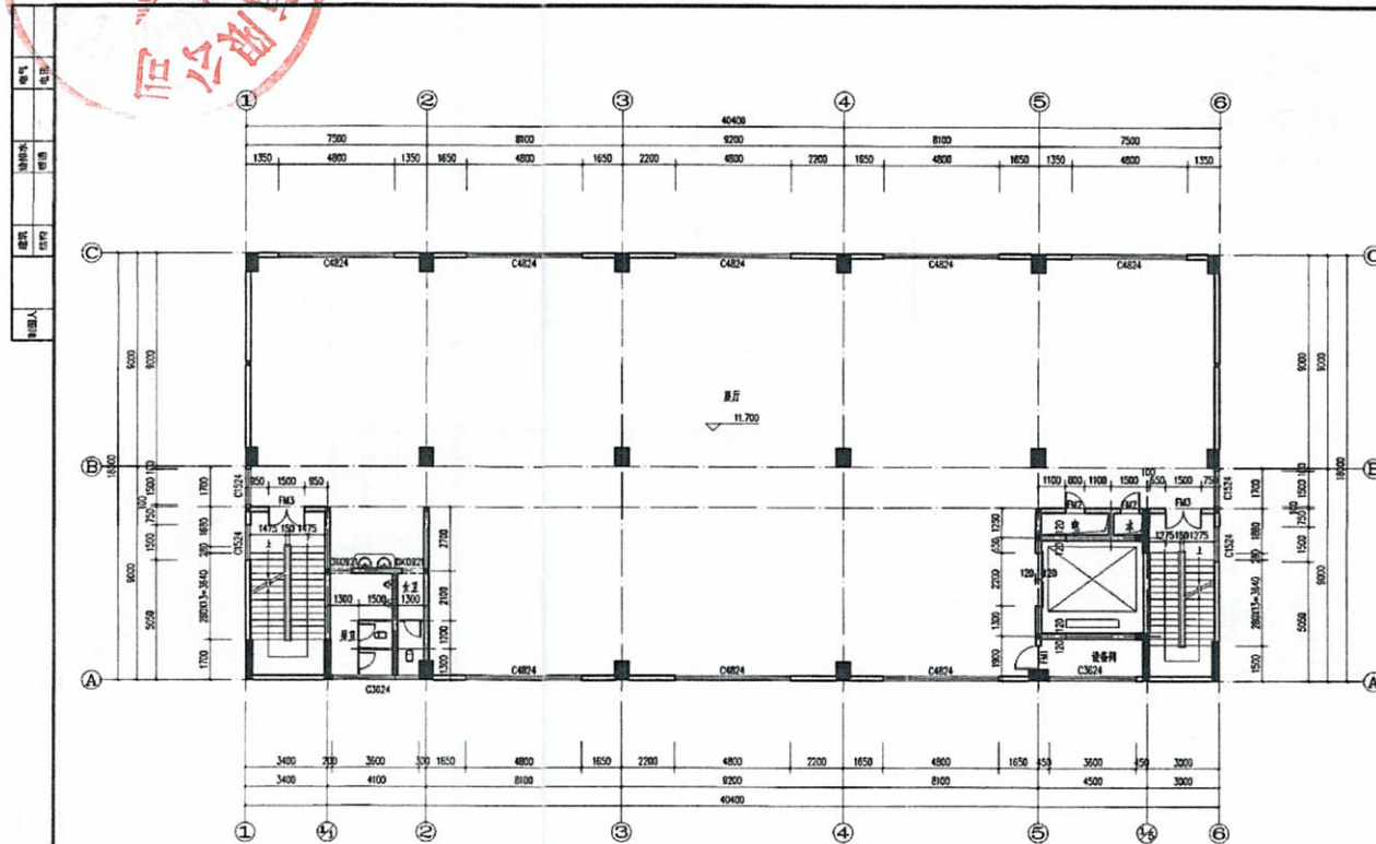
三层平面图 1:100
