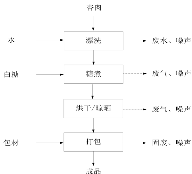
图 2-4 杏肉生产工艺流程图
