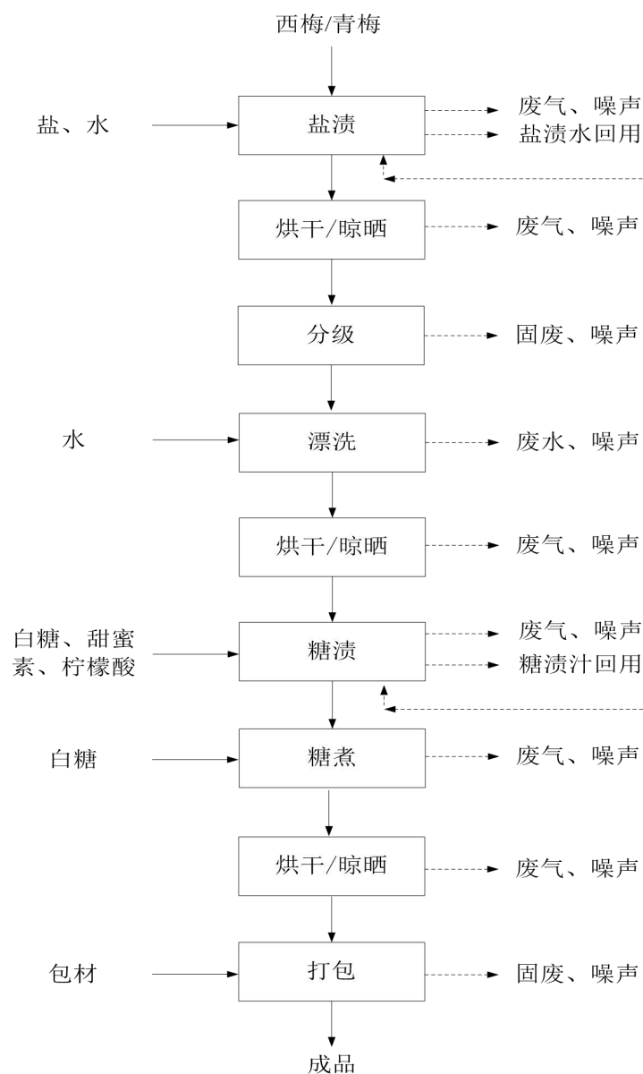
图 2-3 西梅/话梅生产工艺流程图
